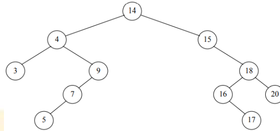
Fig 13.3: Preorder: 14 4 3 9 7 5 15 18 16 17 20
